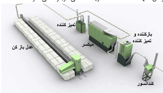
شکل ۱۰ - یک نمونه از خط حلاجی اتوماتیک
