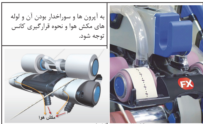
شکل ۲۸- سیستم کامپکت به روش زینسر
