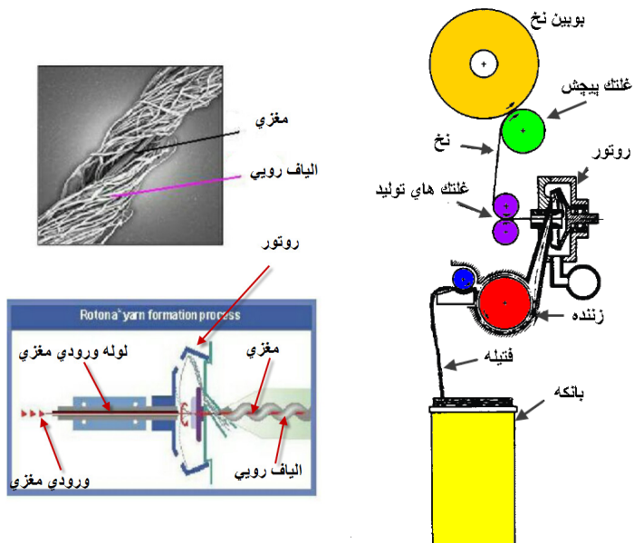
الف - نمای کلی یک واحد روتور ( چرخانه ) ب - نحوه تولید نخ مغزی دار
