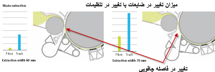
شکل ۳۵- تغییر در چاقویی و اثر آن در ضایعات
