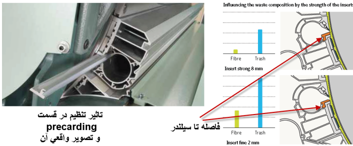
شکل ۳۴- تأثیر فاصله پیش کاردینگ ها
